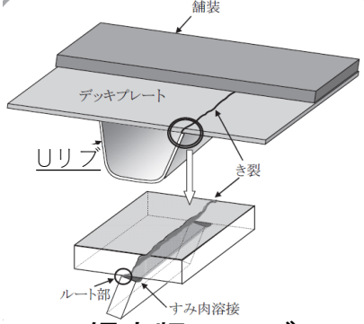
鋼床版のUリブ
