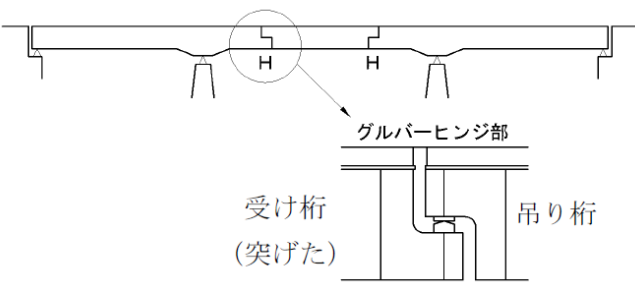
主桁端部 (コンクリート橋)
