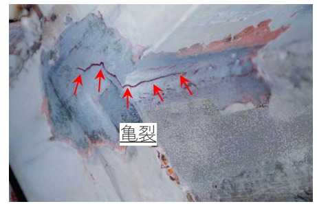
非破壊検査(磁粉探傷検査)
