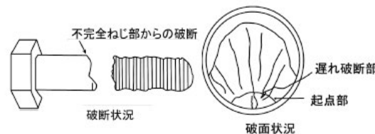
高力ボルト(F11T)の遅れ破壊
